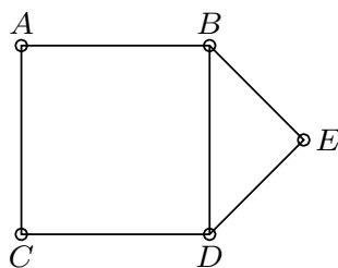
Fig. 29. A graph.
