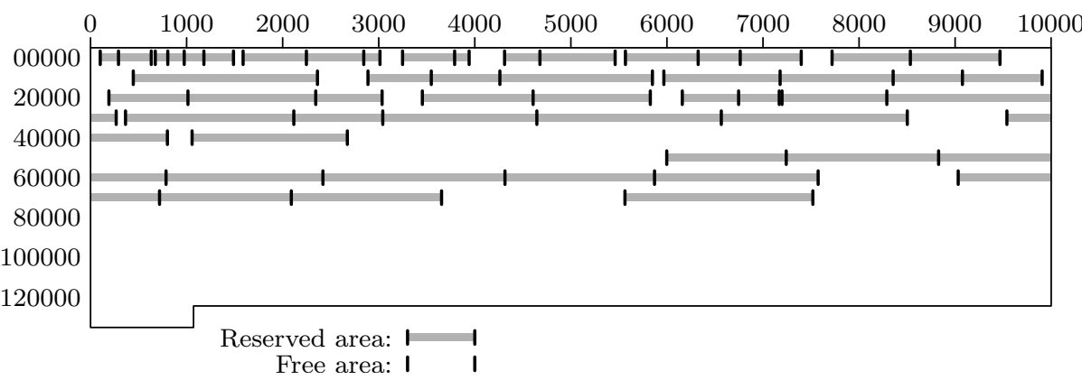
Fig. 42. A memory map.
