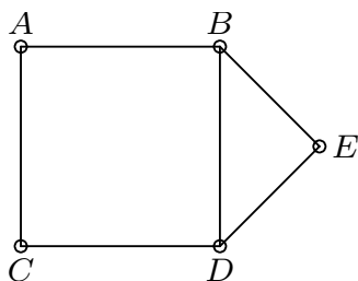
Fig. 29. A graph.
