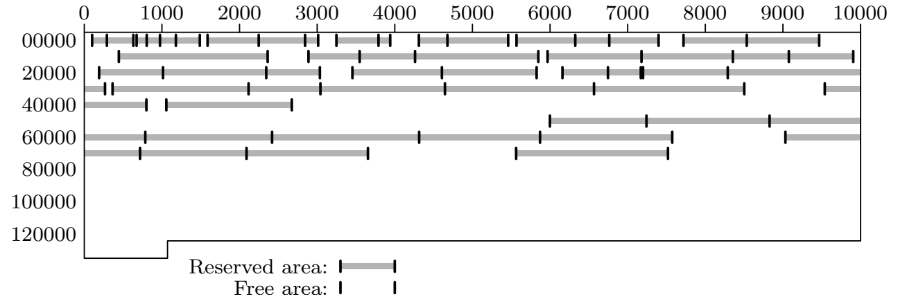
Fig. 42. A memory map.
